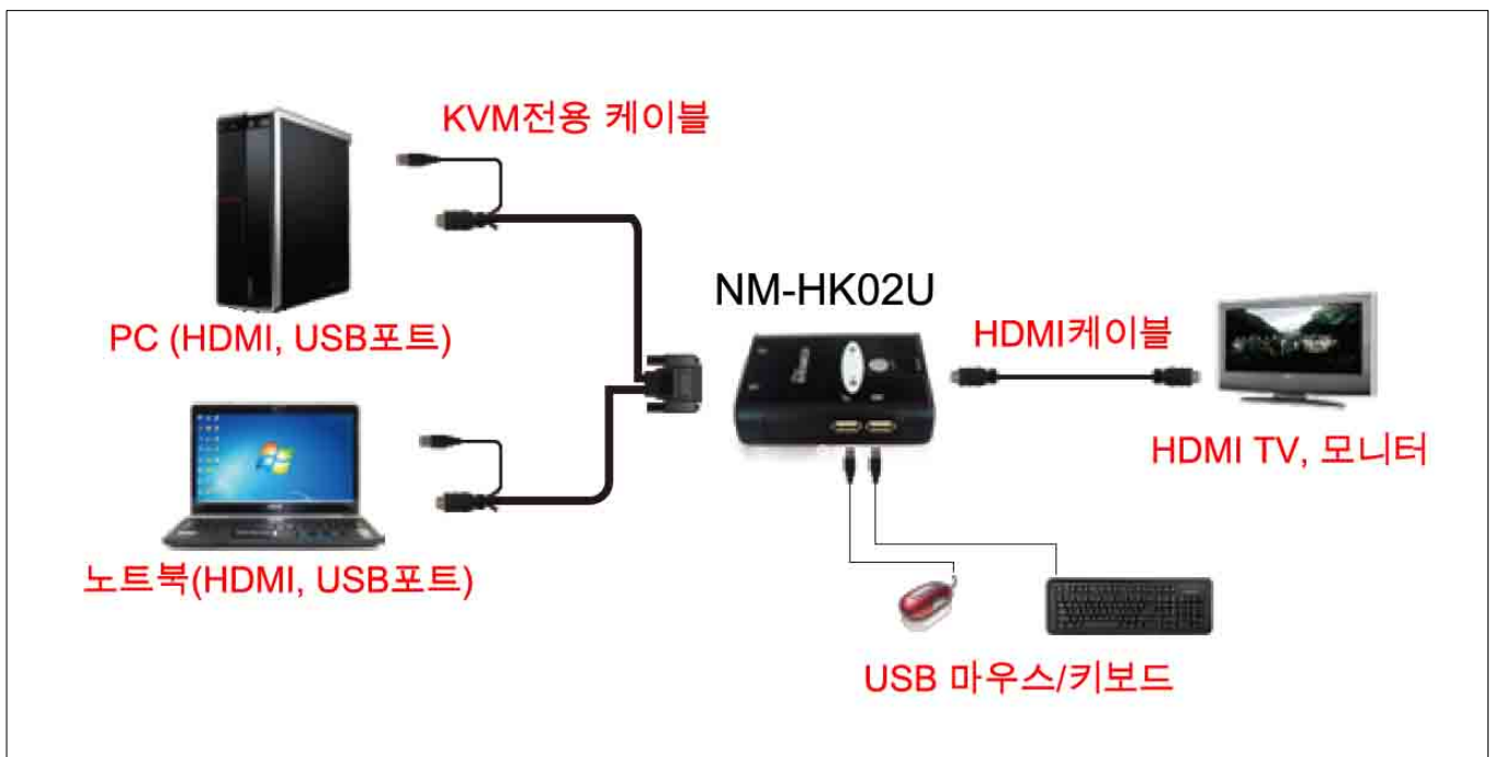
<NM-HK02U 제품 연결도>
